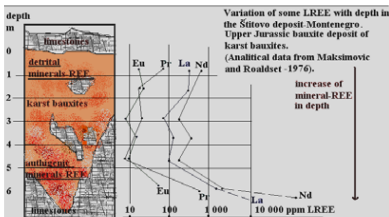
Fig. 1: Esempio di concentrazione di minerali REE autigeni contenuti in bauxite rossa boehmica sul fondo del deposito: Štitovo-Montenegro. Da MAKSIMOVIĆ et ROALDSET (1976).
